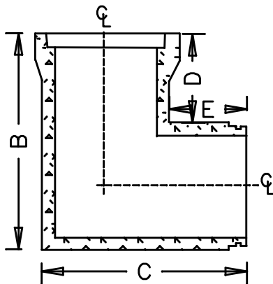
90° Bend
