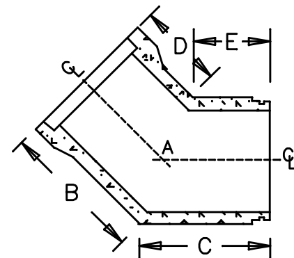
45° Bend
